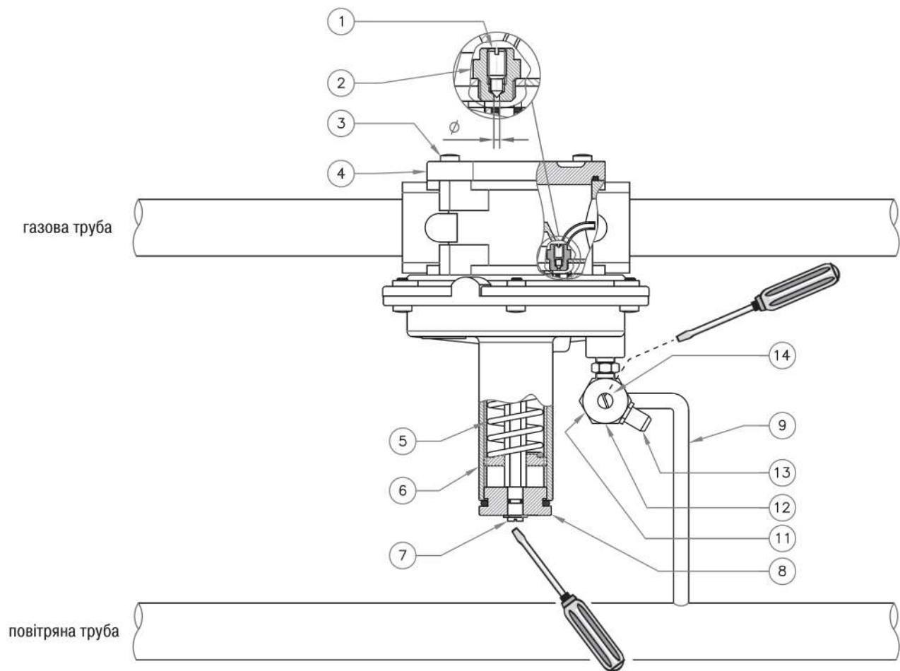
Рис. 2 Співвідношення газ/повітря=1:2 - 1:10
