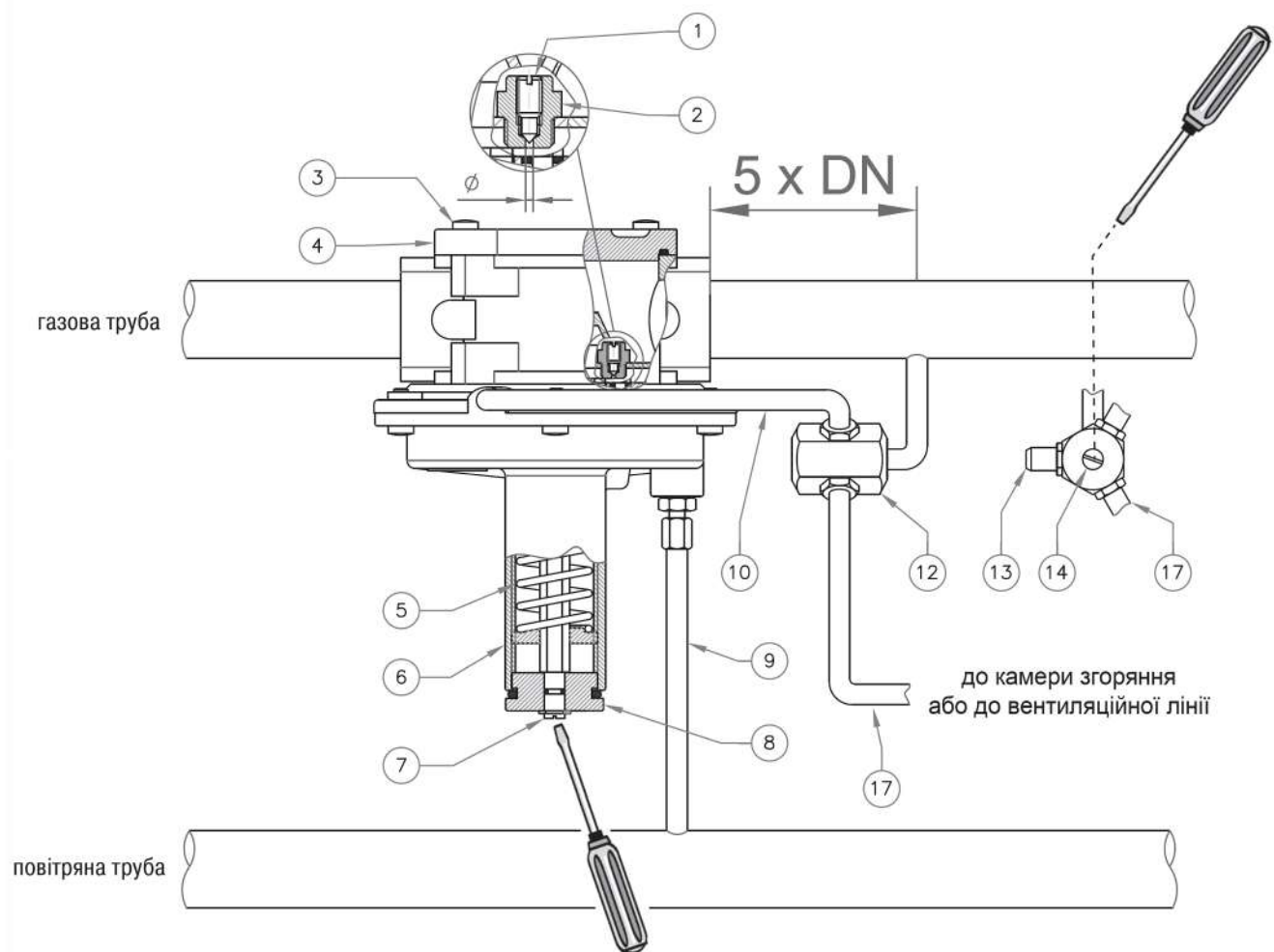
Рис. 3 Співвідношення газ/повітря=2:1 - 10:1
